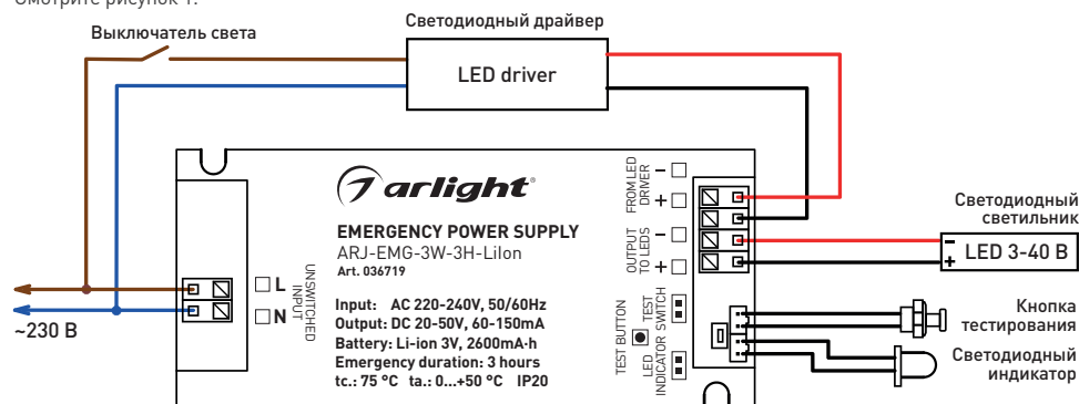
Рисунок 1. Стандартная схема подключения
