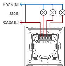
Рис. 3. Схема подключения (0500042,0500048,0500047,0500046)
